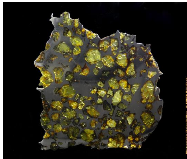
Pallasite de la collection du Musée de Minéralogie, en exposition permanente (#76760 ; 13.6 x 13 x 0.2 cm).
